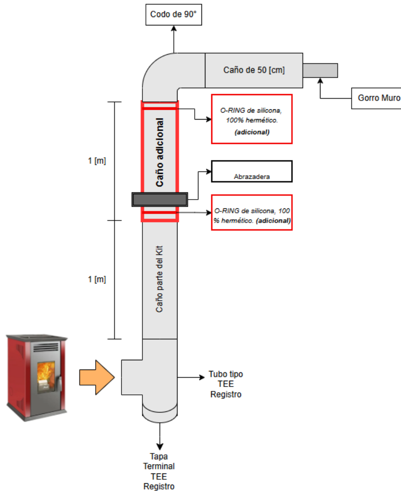
Ilustración 3: Repuestos o componentes requeridos adicionales señalados en color ROJO
