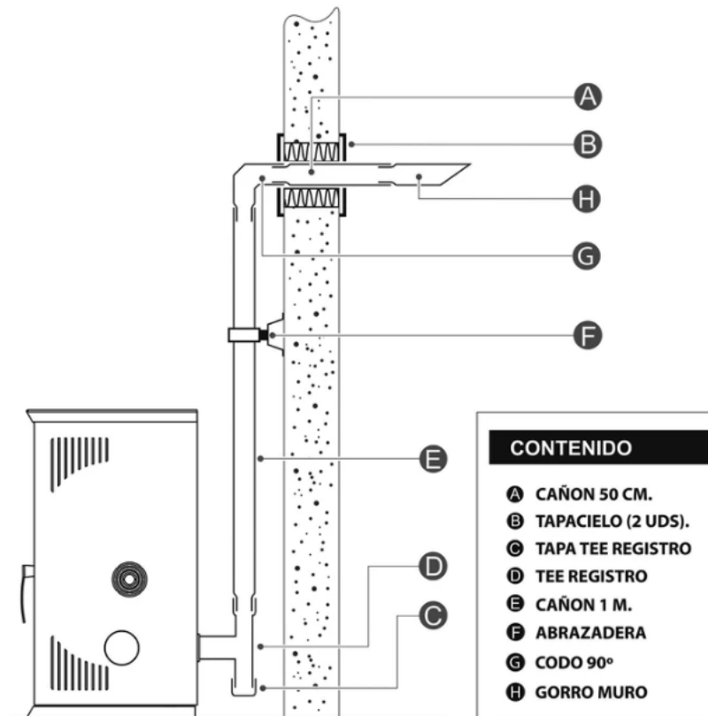
Ilustración 2: Componentes Kit Instalación Amesti. Elemento solicitado en el recuadro N°4
